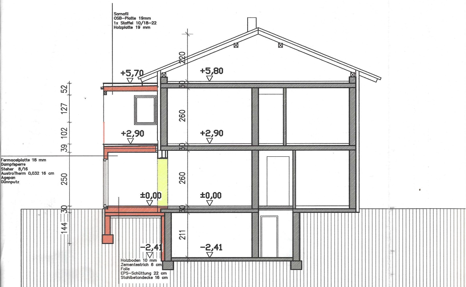
SCHNITT A-A
